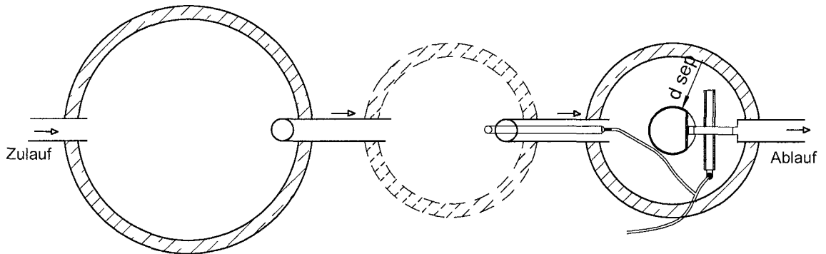
Grobfang/ Schlammsp.
