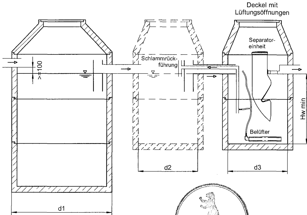
Grobfang/ Schlammsp.
