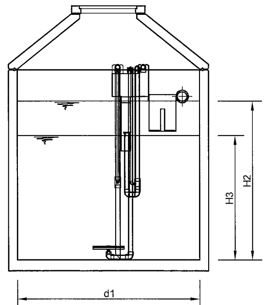
Schnitt C-C
