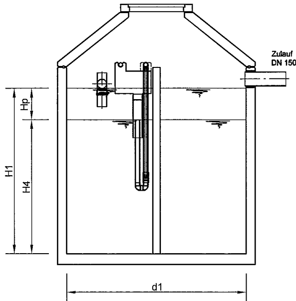
Schnitt A-A
