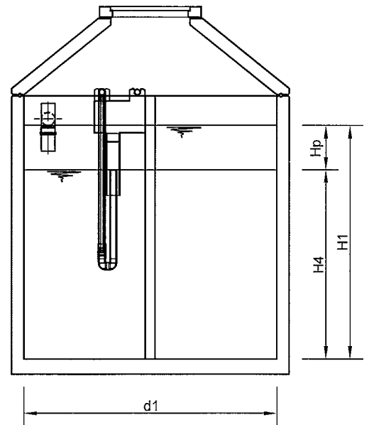
Schnitt C-C
