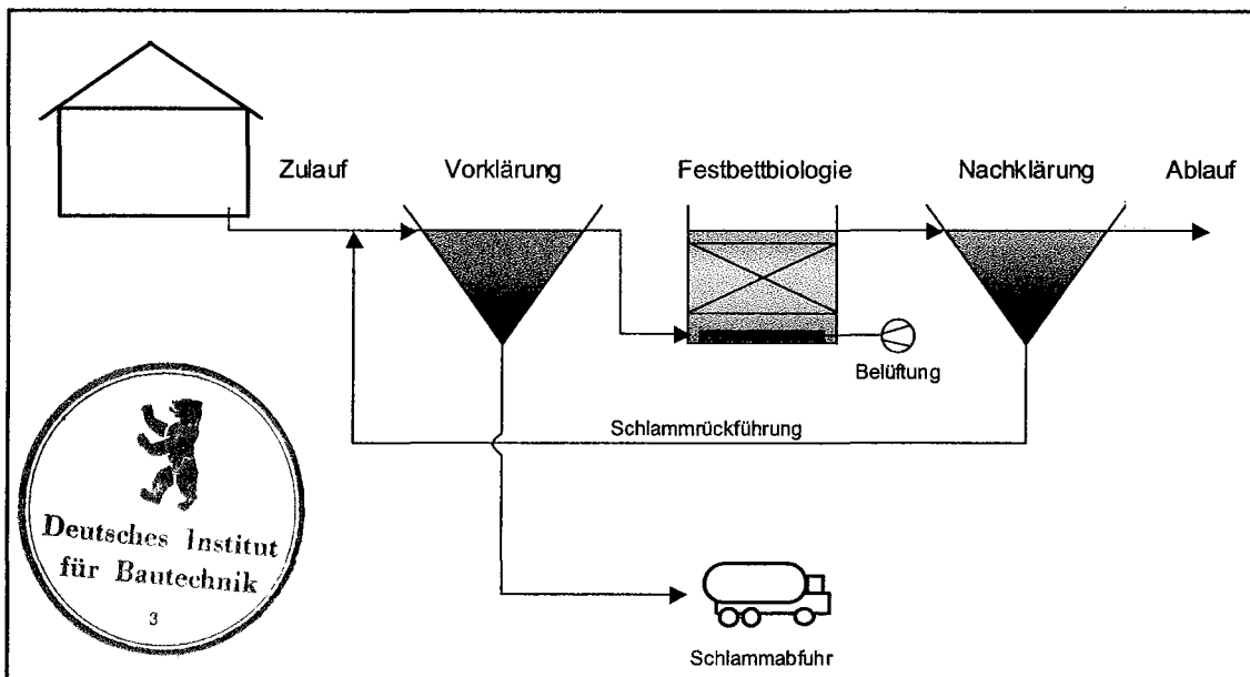
Abbildung 1: Schematische Darstellung der Reinigungsfunktion
