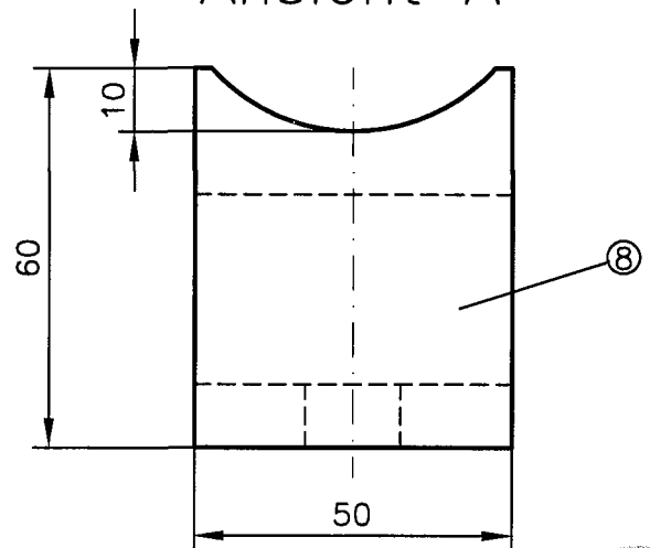
Ansicht A
