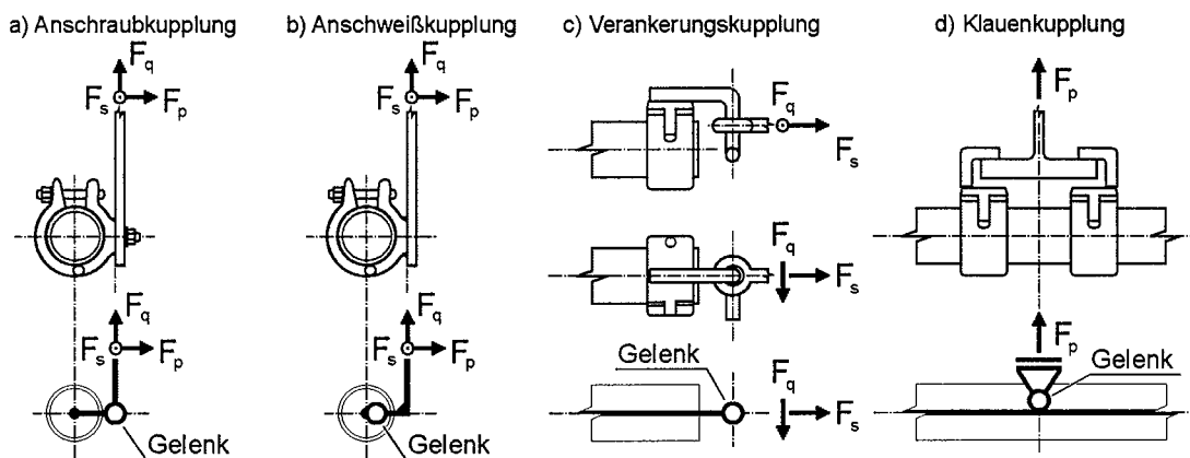
Bild 1a bis d: Statische Systeme der verschiedenen Anschlussvarianten
