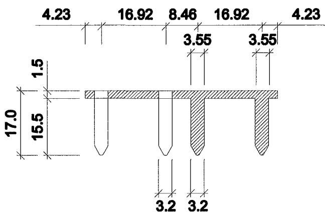
SCHNITT A-A in Querrichtung
