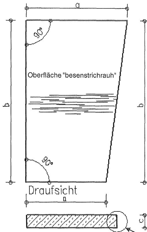
Detail A: Plattenkantenabstufung Passplatte
