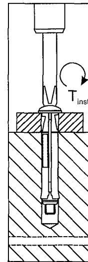
Aufbringen des Drehmoments T_{inst}
