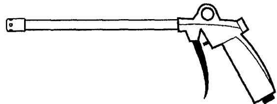
Empfohlene Druckluftpistole (min 6 bar) Bohrerdurchmesser ( d_0 ): 10 mm bis 37 mm
