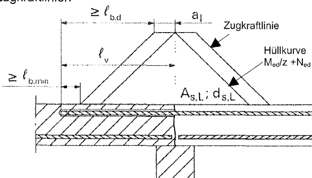
Bild 5: Verankerung von Bewehrung zur Deckung der Zugkraftlinien
