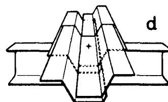
Verbindung mit einem Längs- und Querstoß
