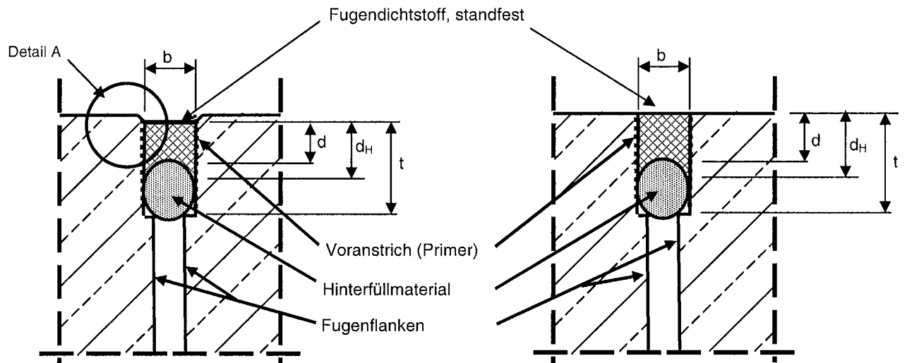
Befahrbare Fugenkonstruktion
