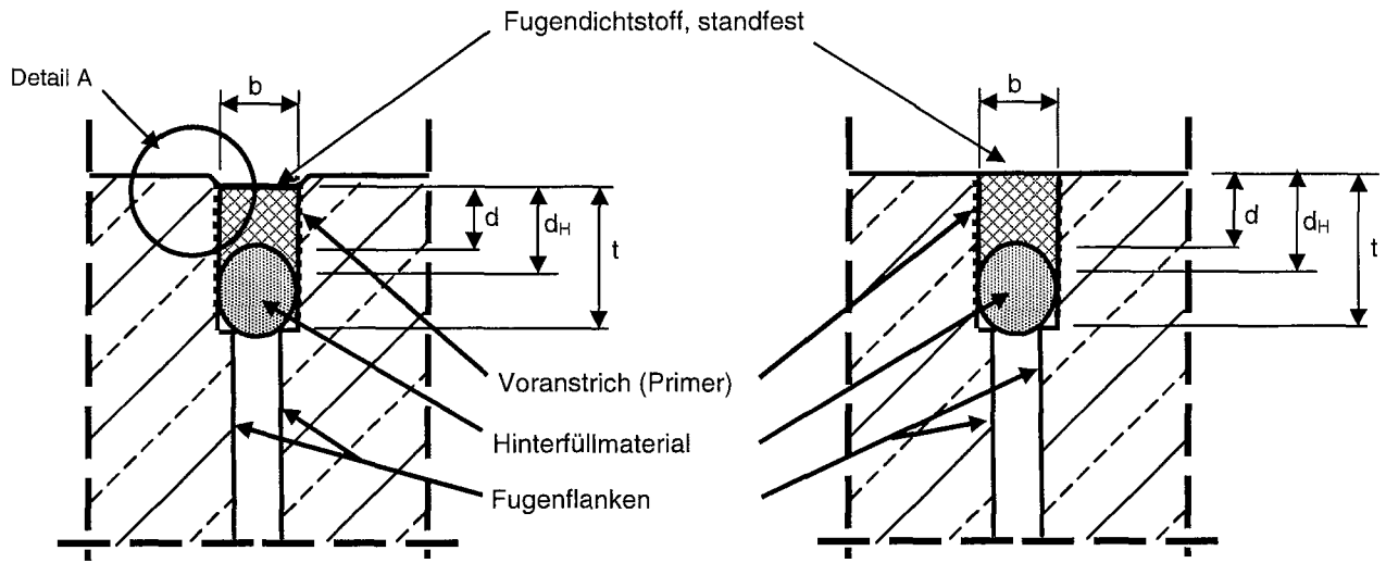
Befahrbare Fugenkonstruktion
