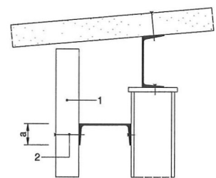
Bild 6 Traufpunkt
