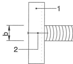
Bild 2 Holz- Auflager
