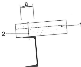
Bild 4 Traufpunkt
