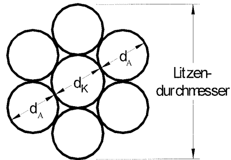
Bild 1 : Litzenquerschnitt
