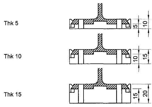
Thermokappen
