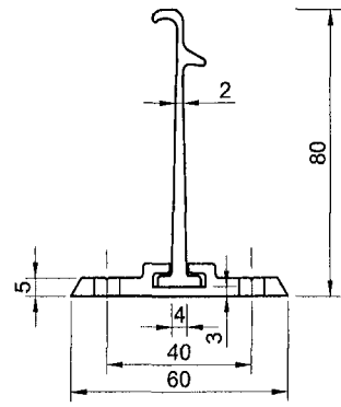
Gleithalter
