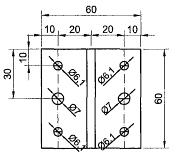
Thermokappen
