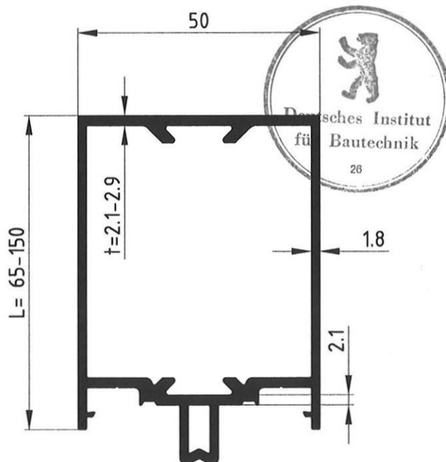
Tragprofil 50mm Bautiefe: 65mm bis 150mm
