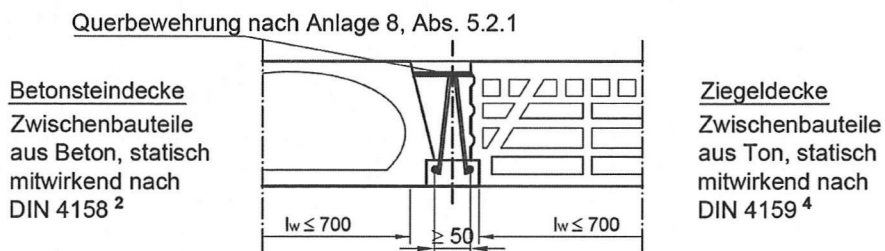
Bild 6: Rippendecke nach Anlage 8, Abschnitt 5
