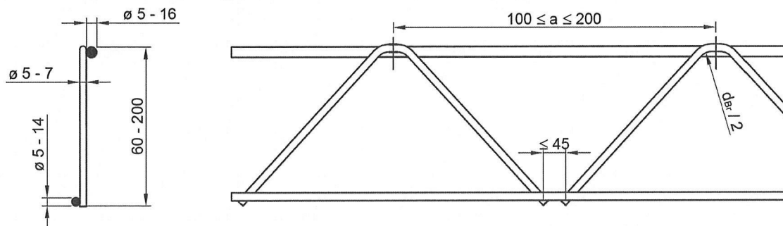
Bild 3: DH-Gitterträger
