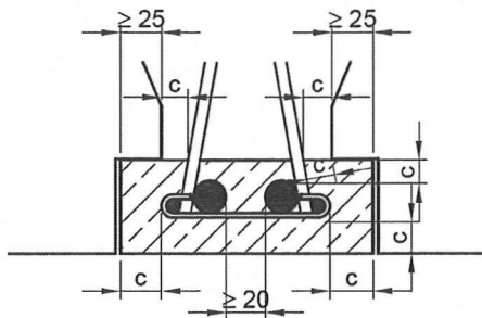
Bild 12: D- / E-Träger mit Betonfußleiste und Querbügeln
