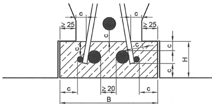
Bild 11: Betonfußleiste mit D- bzw. E-Träger und Zulagestäben
