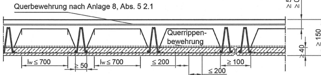
Bild 11: Betonfußleiste mit D- bzw. E-Träger und Zulagestäben
