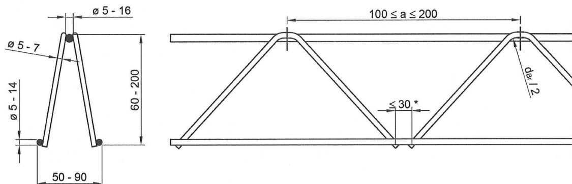
Bild 1: D-Gitterträger
