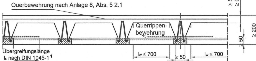
Bild 9: Rippelementdecke mit Betonschalung nach Anlage 8, Abschnitt 5
