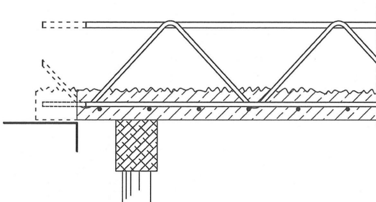
Bild 20: Auflagerung mit Montageunterstützung am Rand
