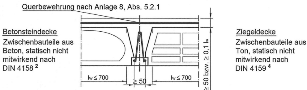
Bild 7: Rippendecke nach Anlage 8, Abschnitt 5
