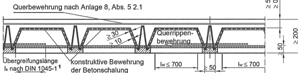
Bild 9: Rippelementdecke mit Betonschalung nach Anlage 8, Abschnitt 5
