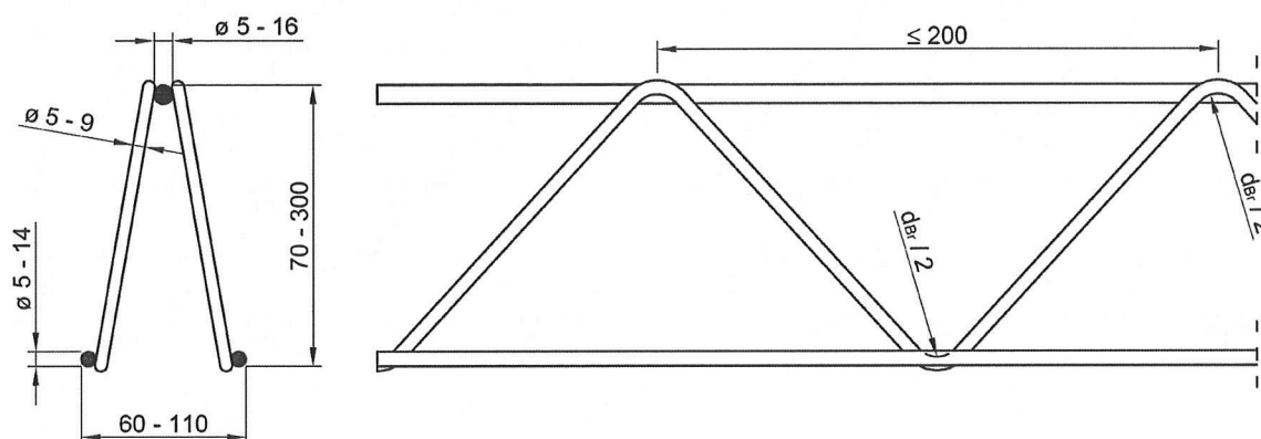
Bild 2: E-Gitterträger
