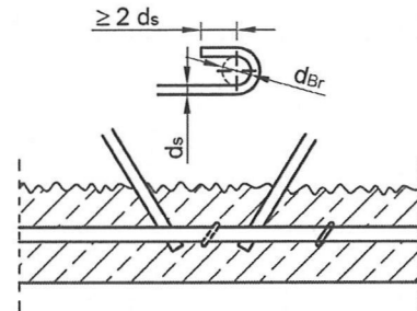
Bild 13: Querbügel
