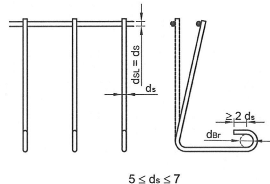
Bild 17: D- / E-Träger mit Betonfußleiste und zweischschnittigen Bügel
