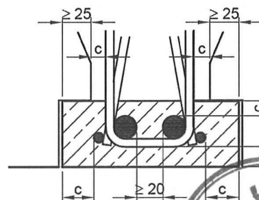
Bild 17: D- / E-Träger mit Betonfußleiste und zweischschnittigen Bügel
