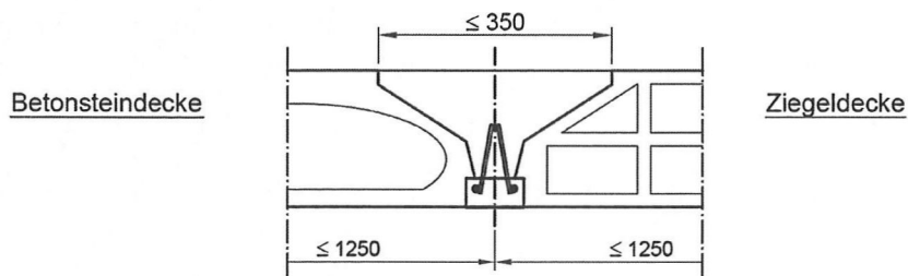
Bild 5: Rippendecke nach Anlage 8, Abschnitt 5
