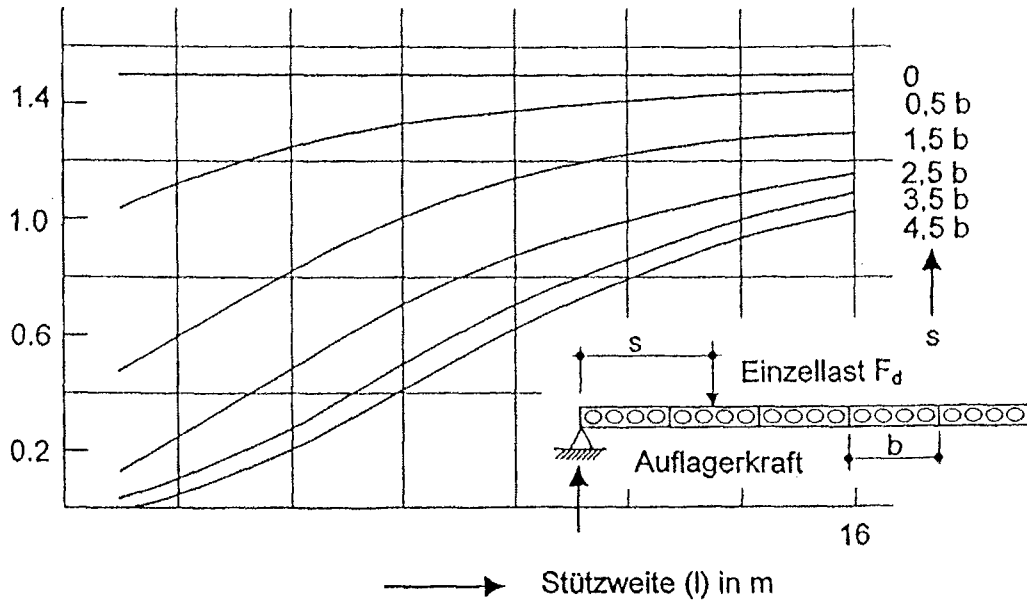
Auflagerkraft am Längsrand infolge Einzellast in Feldmitte
