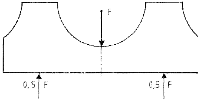
Bild 1: Belastungsanordnung Biegeversuch
