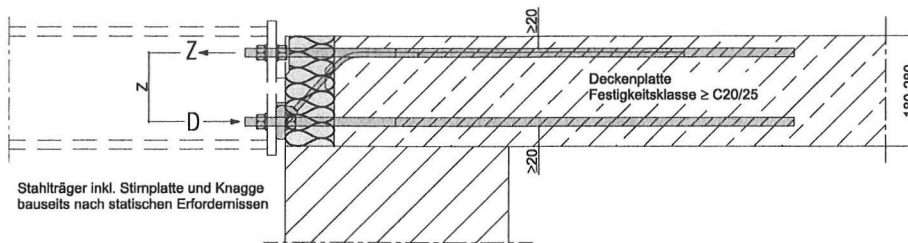
Abb. 11: Schöck Isokorb Typ KS14 VV
