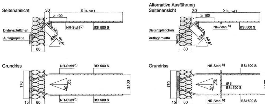
Abb. 14a bis 14d: Querkraftstäbe 2 Ø 8 inkl. Auflagerplatte
