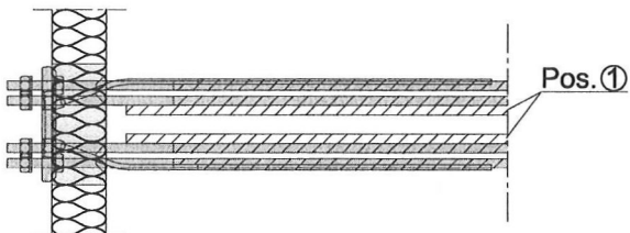
Abb. 47 Draufsicht: Schöck Isokorb Typ KS14 VV
