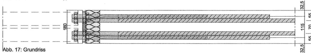
Abb. 17: Grundriss
