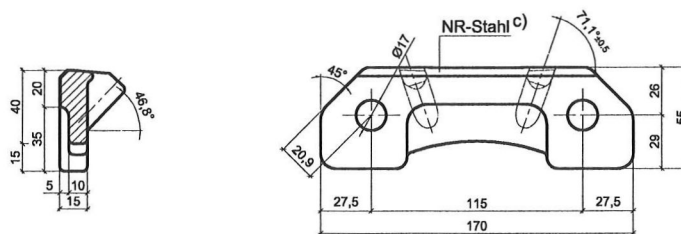
Abb. 10: Auflagerplatte
