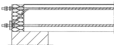
Abb. 46 Seitenansicht: Schöck Isokorb Typ KS14 VV
