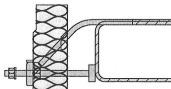
Abb.4 Schöck Isokorb Typ QS10 und QS12
