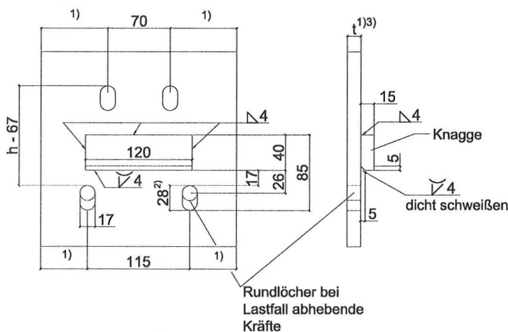
Abb. 39 Bauseitige Stirnplatte zu Schöck Isokorb Typ KS14 V8, KS14 V10 und KS14 VV
