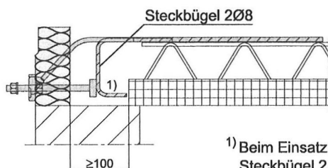
Abb. 49 Bauseitige Anschlussbewehrung für Schöck Isokorb Typ QS
