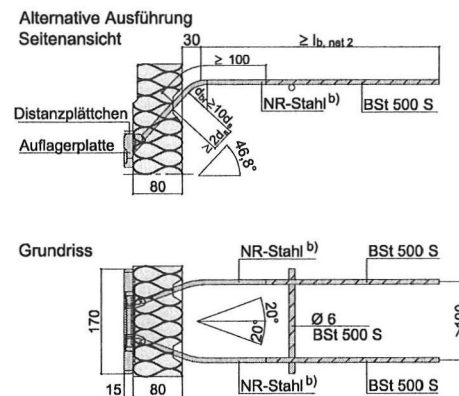
Abb. 8: Drucklager 2 Ø 14
