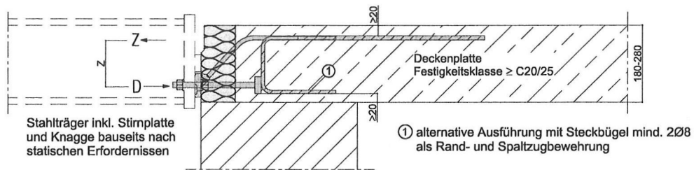
Abb. 22: Schöck Isokorb Typ QS10 und QS12
