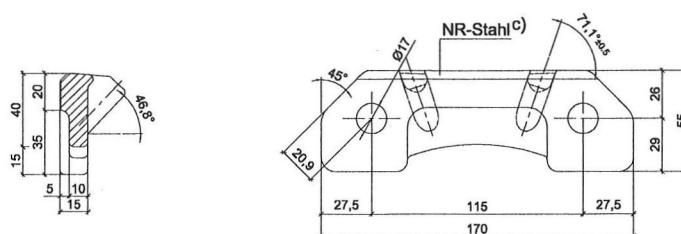
Abb. 15: Auflagerplatte
