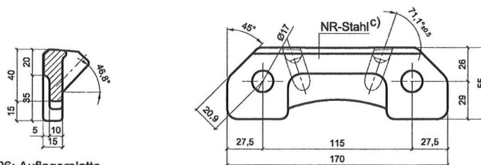
Abb. 26: Auflagerplatte
