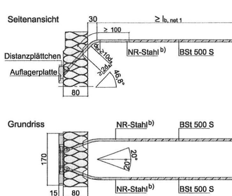
Abb. 9a bis 9d: Querkräfte 2 Ø d s inkl. Auflagerplatte
