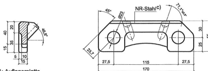
Abb. 21: Auflagerplatte
