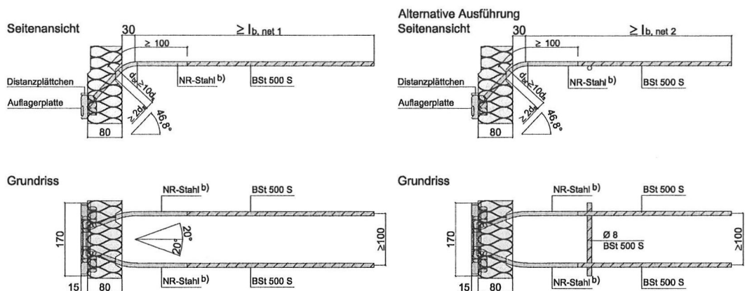
Abb. 25a bis 25d: Querkraftstäbe 2 Ø d_s inkl. Auflagerplatte
