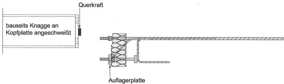
Abb. 36 Querkraftübertragung durch Knagge
