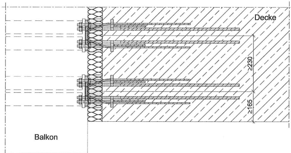
Abb. 35 Achs- und Randabstände
