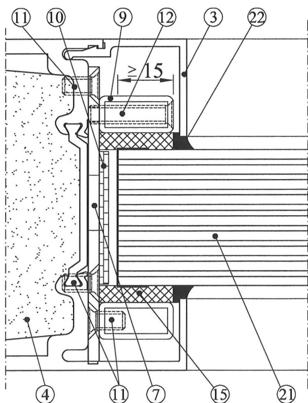
Scheibe "Pilkington Pyrostop -Typ 90-1.." "Pilkington Pyrostop -Typ 90-2.."
