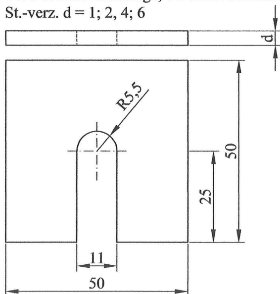
Zwischenlage für Rahmenbefestigung, Pos. (18) bzw. Pos. (19)
