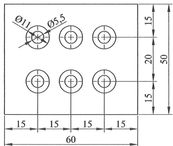
Ankerplatte, Pos. (43) 4 mm St.-Blech, verz.
