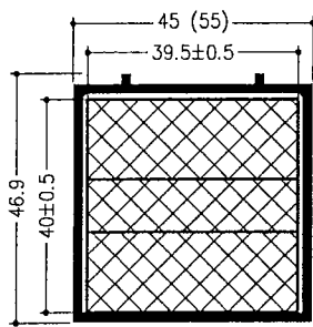
Einschubprofil
