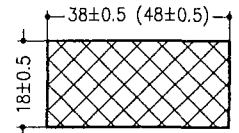
Brandschutzstreifen Gipsfaserplatte
