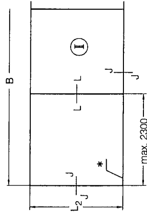
Liegendes Dach
