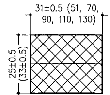
Brandschutzstreifen Gipsfaserplatte
