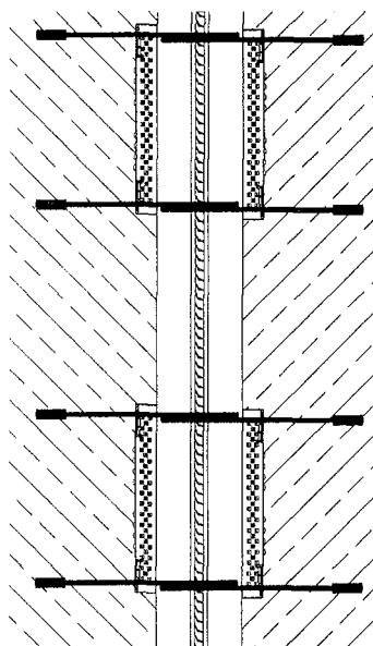
Bild 9: Regeldetail Schlaufenüberlappung
