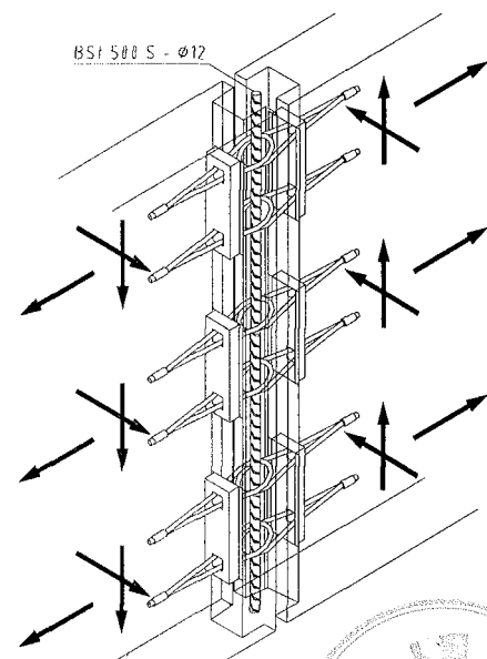
Bild 16: Kombinierte Beanspruchung
