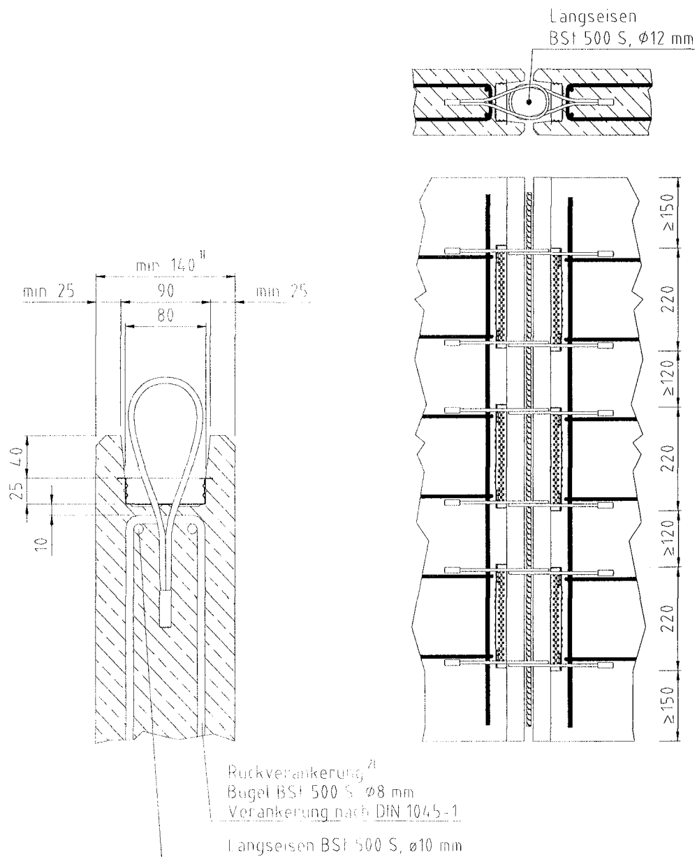
Bild 7: Vergussnut, Bewehrung
