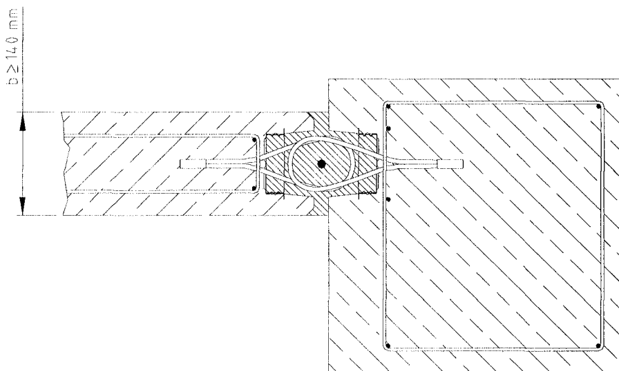
Bild 4: Stützen - Wandverbindung
