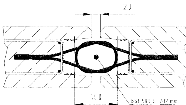
Bild 8: Regelfall Fuge
