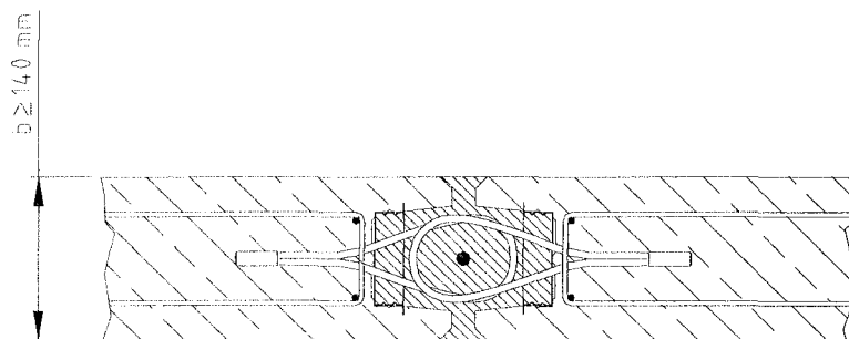
Bild 3: Wand - Wandverbindung
