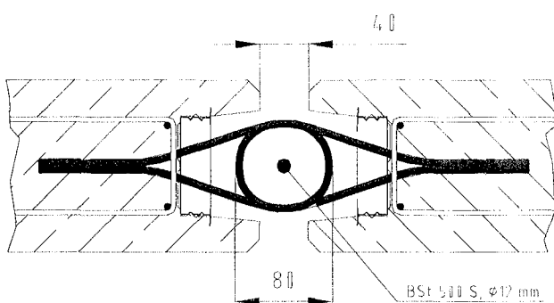
Bild 11: Maximale Fugenbreite
