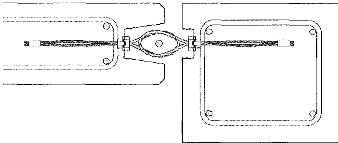
Bild 15: Anschluss Wand – Stütze
