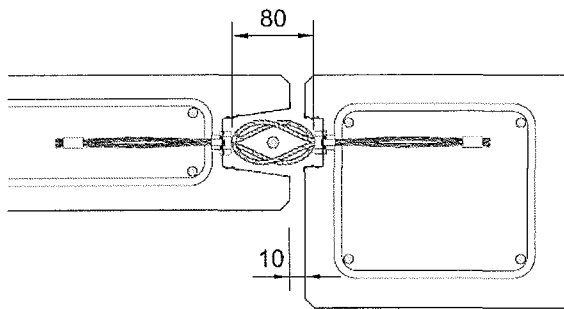
Bild 10: Minimalfuge
