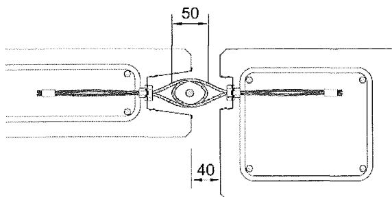
Bild 11: Maximalfuge
