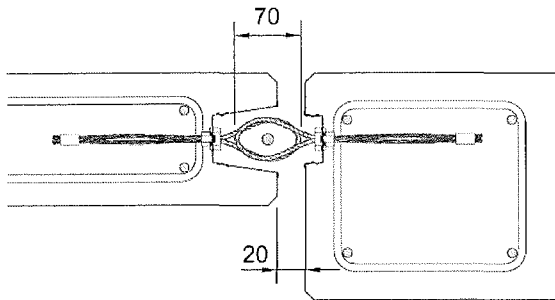
Bild 8: Horizontale Solllage
