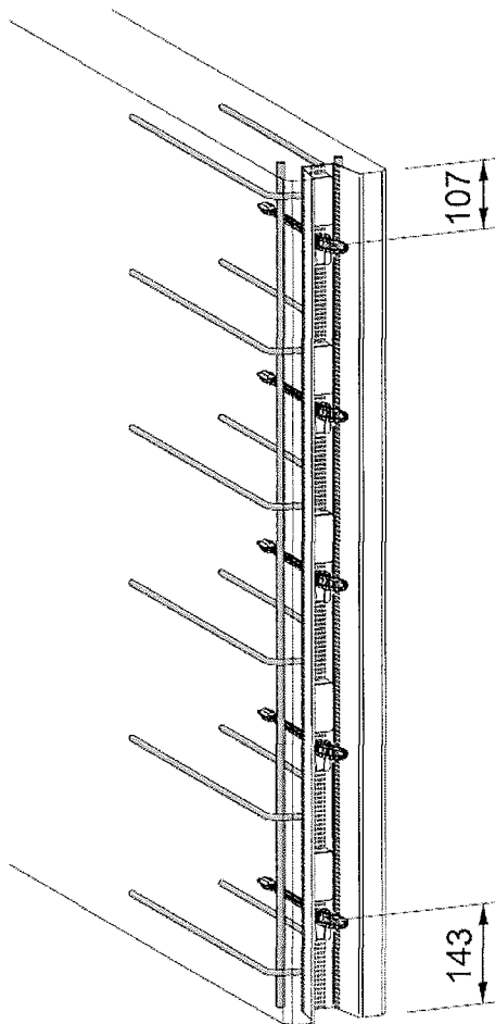
Bild 6: Randabstände
