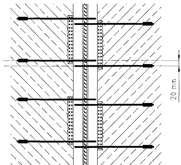
Bild 14: Maximale vertikale Fehllage: 20 mm
