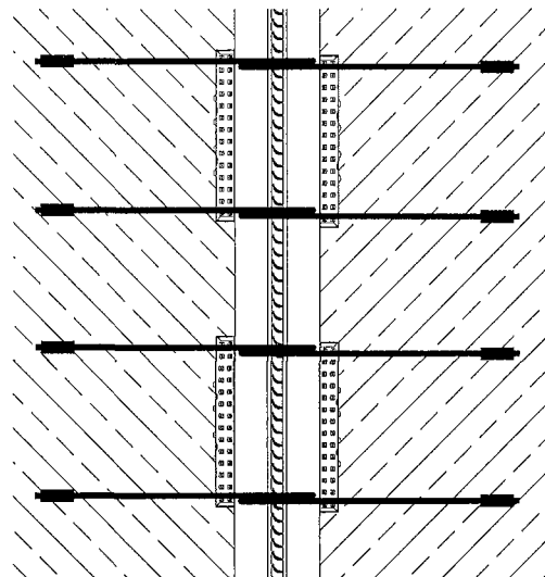
Bild 13: Regelfall Schlaufenüberlappung
