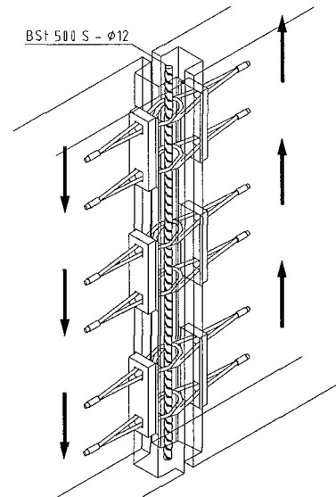
Bild 16: Beanspruchung parallel zur Fugenlängsrichtung
