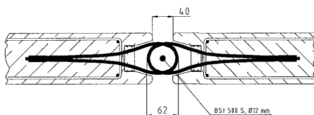
Bild 12: Maximale Fuge
