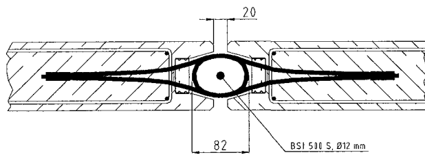
Bild 10: Regelfall Fuge
