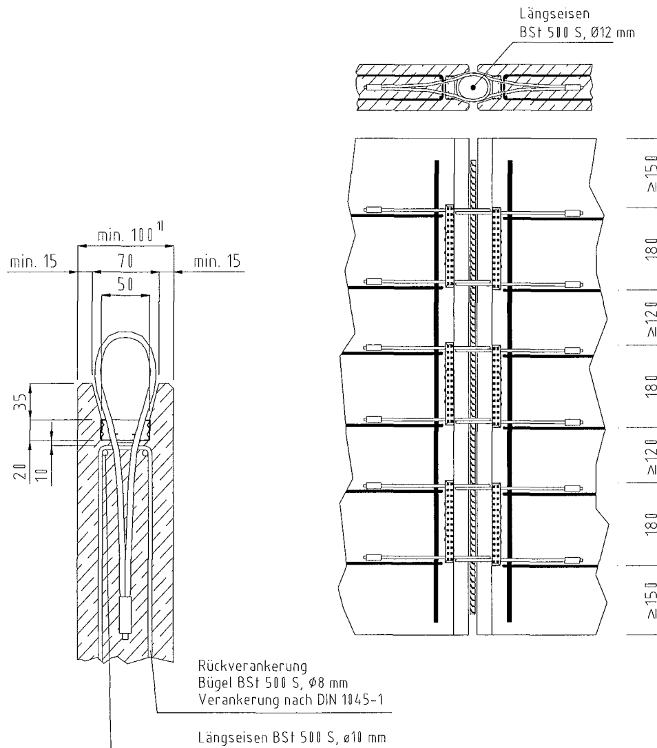
Bild 9: Vergussnut, Bewehrung
