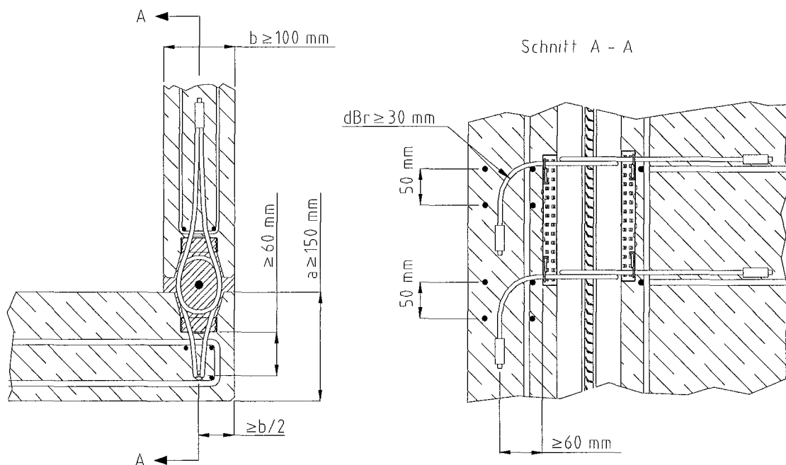
Bild 6: Wand – Wand – Eckverbindung - Detail mit abgewinkelten Seilschlaufen
