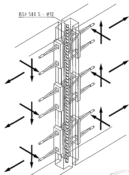
Bild 18: Kombinierte Beanspruchung
