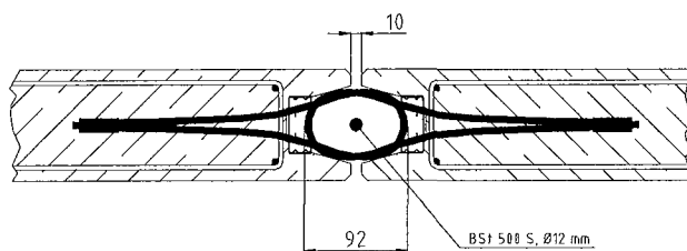
Bild 11: Minimale Fuge
