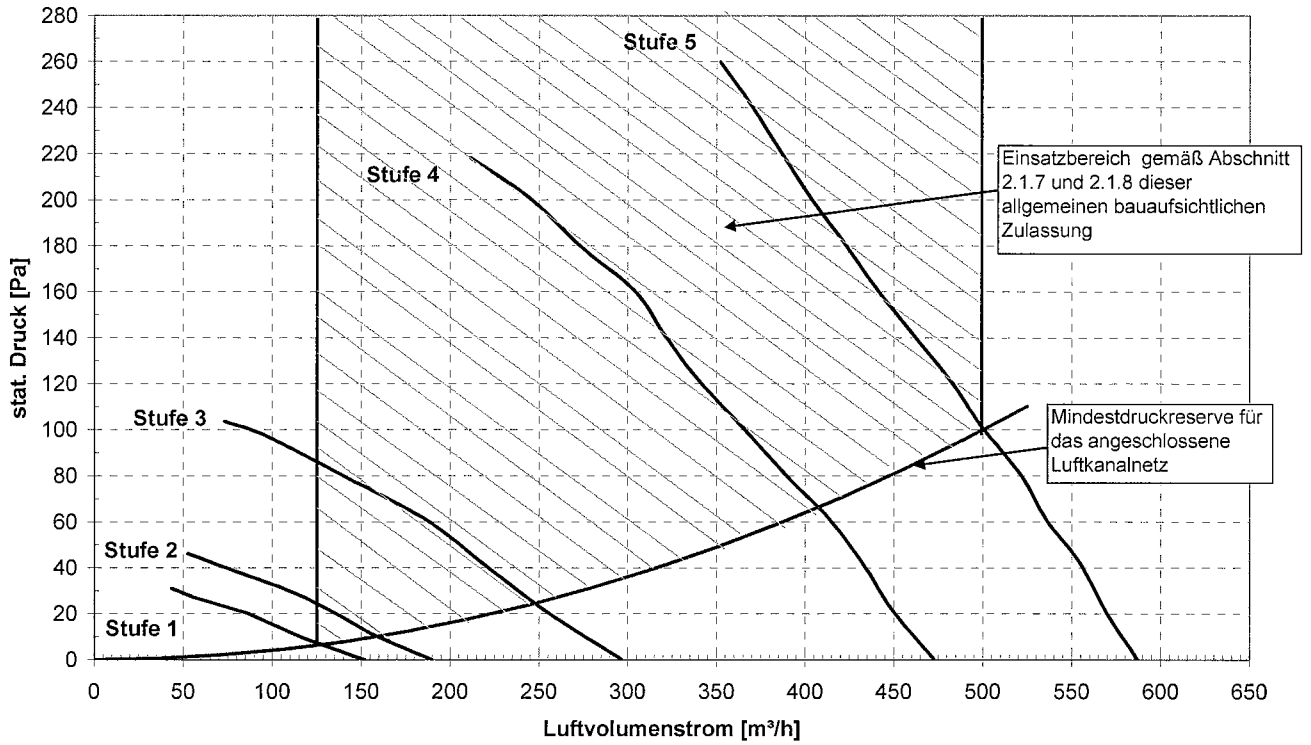
\Delta p, V -Kennlinien Ab-/Fortluft
