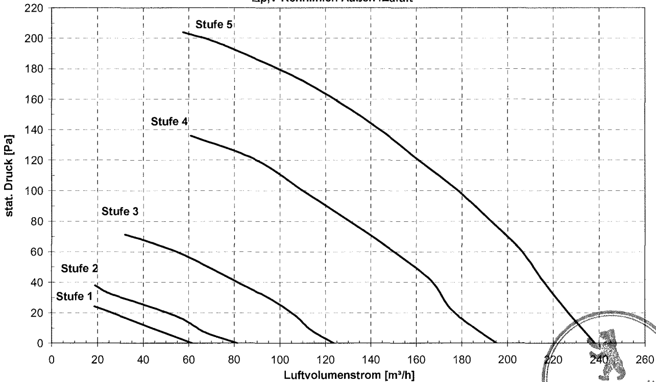
\Delta p, \dot{V} -Kennlinien Außen-/Zuluft
