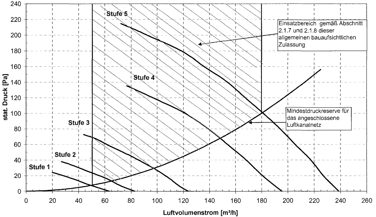
\Delta p, \dot{V} -Kennlinien Ab-/Fortluft
