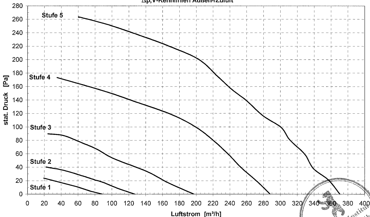
\Delta p, V -Kennlinien Außen-/Zuluft
