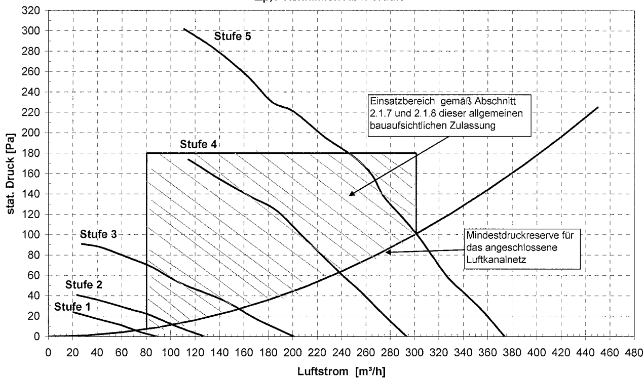
\Delta p, V -Kennlinien Ab-/Fortluft
