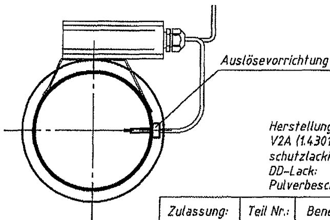
Schnitt A-A
