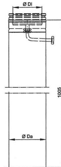
Fußteil Bodenmontage mit Kondensatablauf
