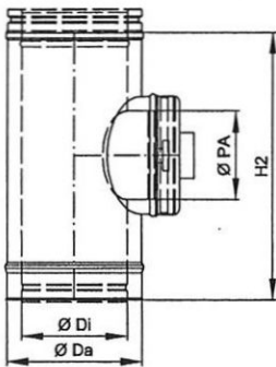
Putztüranschluss (Überdruck)
