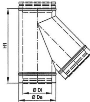
Rauchrohranschluss 45°
