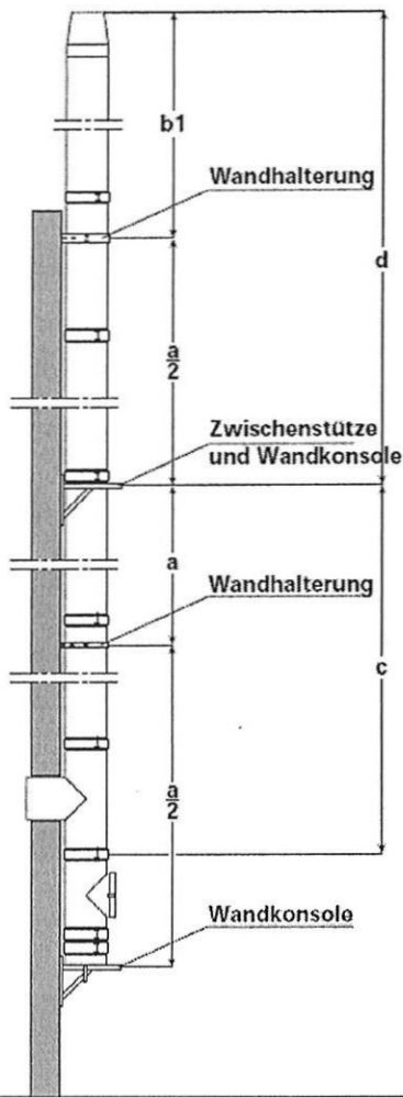
Maximale Höhen in m
