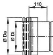
Anschlußübergang DW-EW
