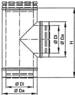
Rauchrohranschluss 90° / 85°
