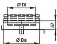
Grundplatte gedämmt mit Kondensatablauf
