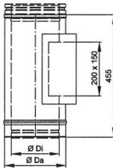
Putztüranschluss (Unterdruck)
