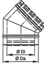
Bögen 15°, 30°, 45°, 85°, 90°
