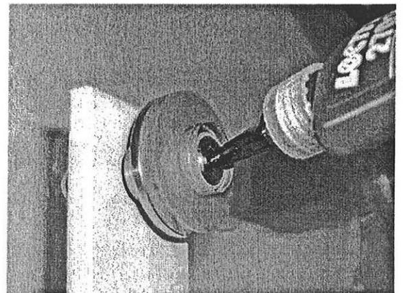
Bild 4: Schraubensicherung anbringen
