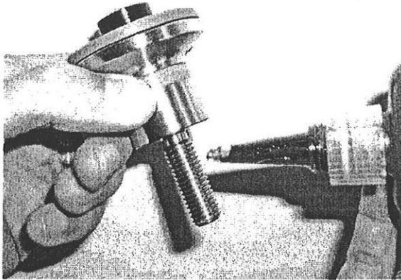
Bild 1: Schraubensicherung anbringen
