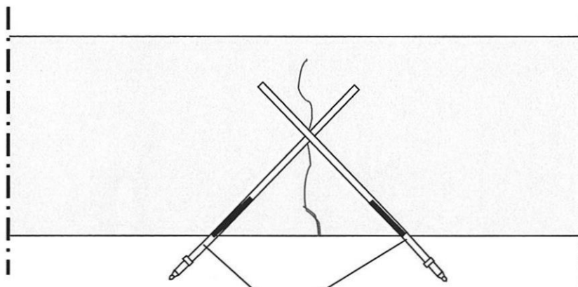
Stahlpacker mit Sollbruchstelle bzw. Sollentnahmestelle 1) und dünner Dichtungsmanschette
