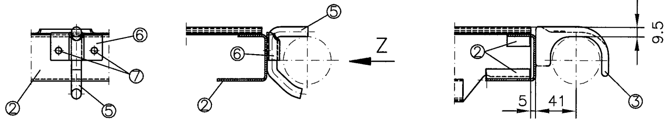
Ansicht Z
