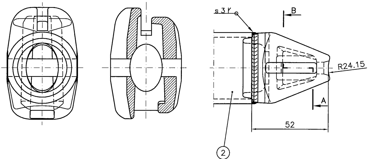
Ansicht X
