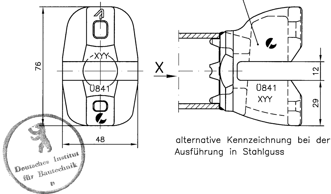
Ansicht X
