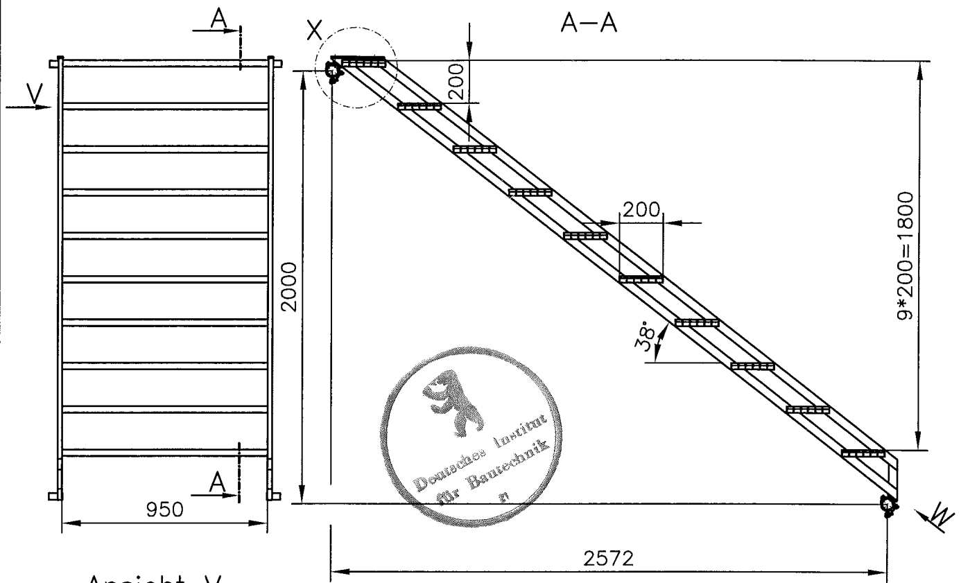
Ansicht V
