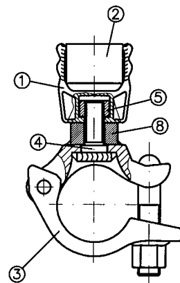
Ansicht A
