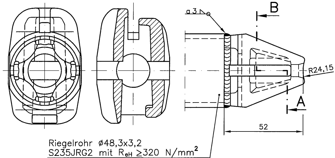
Ansicht X
