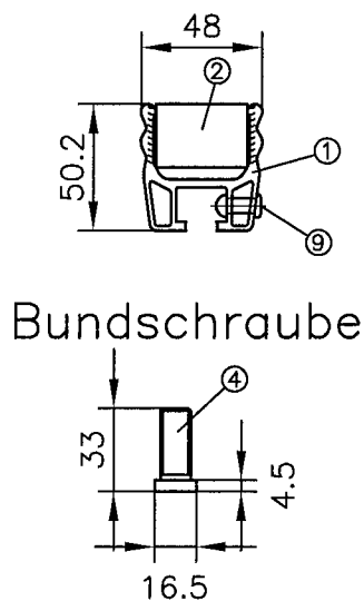
Ansicht C
