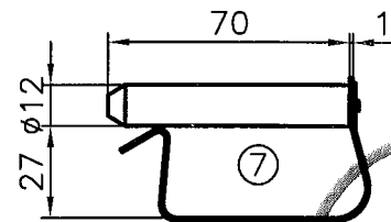
Federsteckbolzen KSB55
