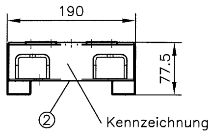
Kopfbeschlagn
