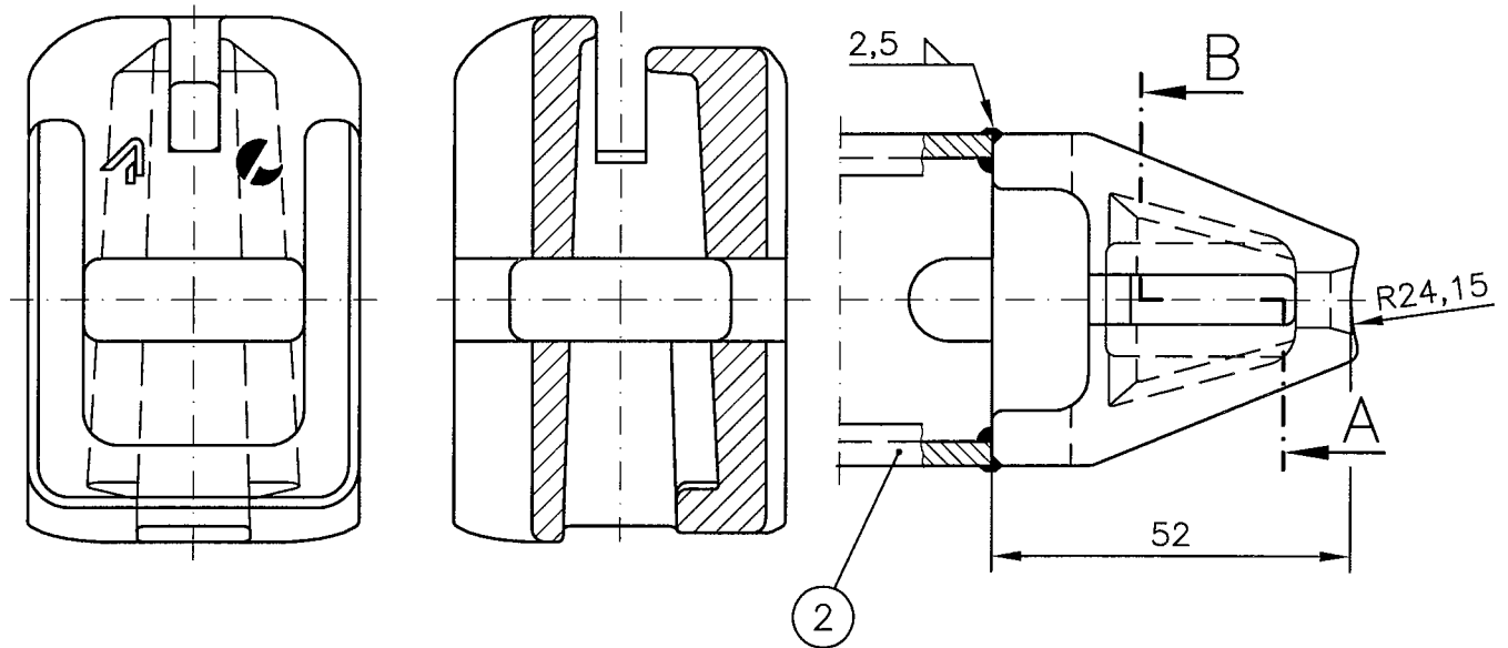
Ansicht X
