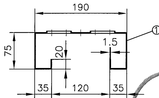
Querschnitt
