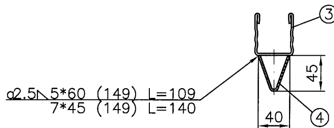
Schnitt A-A
