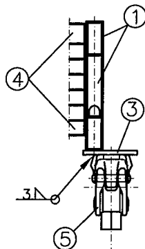
Ansicht W
