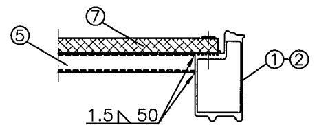
Schnitt B-B
