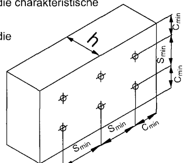
Schema der Dübelabstände
