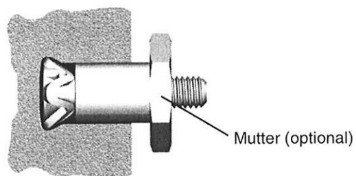
Abstandsmontage (Stahlhülse)
