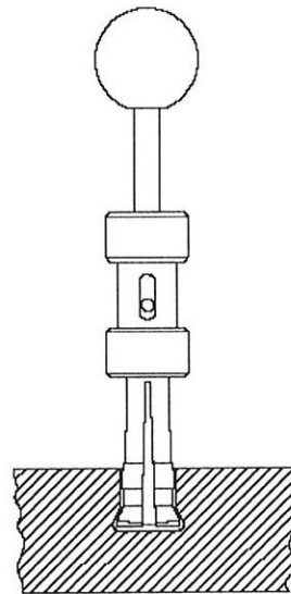
Hinterschnitt-Mindestvolumenlehre
