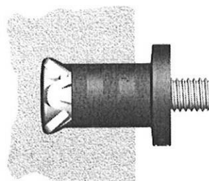
Abstandsmontage (Carbonhülse)
