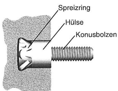
Bündigmontage (Stahlhülse)
