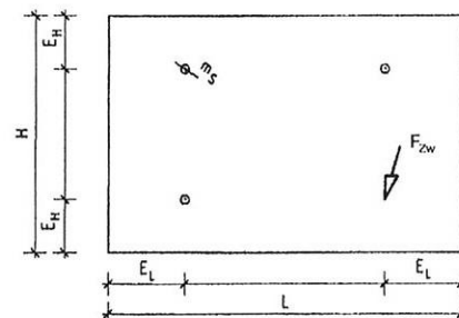
Bild 10: Moment aus Zwangungslast F_{Zw} bei gleichmäßiger Lagerung (Platte ist 3-Punkt gelagert)
