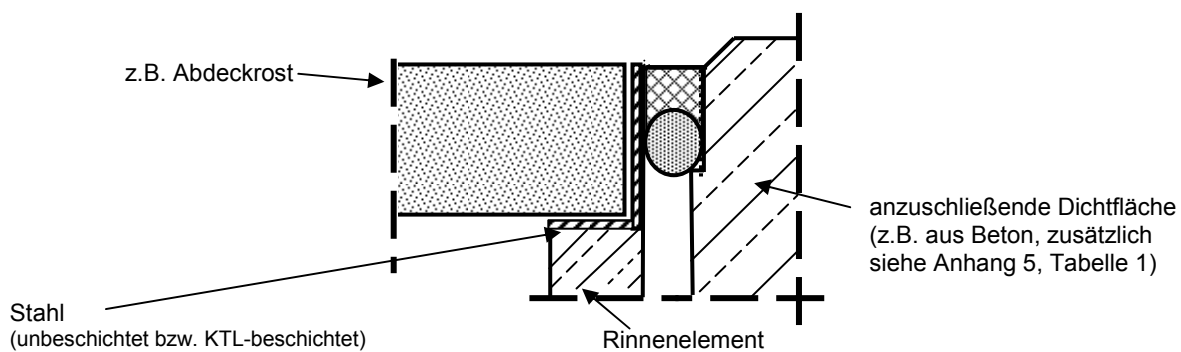
Bild 2: Stahl (unbeschichtet bzw. KTL-beschichtet 1) )
