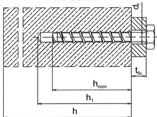
TAPCON-II
