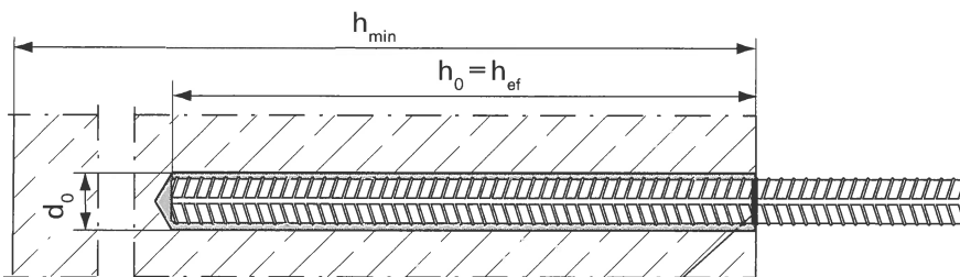
Betonstahl
