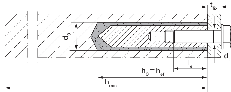
Innengewindeanker UVT Top I Nur Vorsteckmontage
