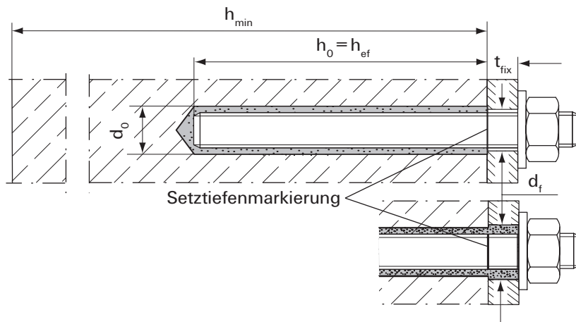
Ankerstangen UVT Top A Vorsteckmontage
