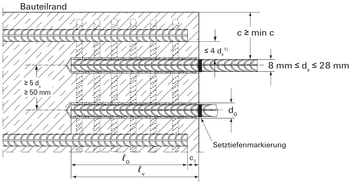
Bild 10: Einbau Bewehrungsanker BRA (Beispiel: Ausführung Glattschaft)
