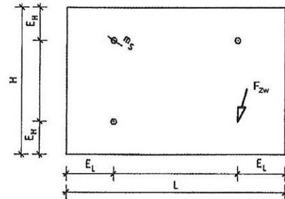
Bild 10: Moment aus Zwängungslast F_{zw} bei gleichmäßiger Lagerung (Platte ist 3-Punkt gelagert)
