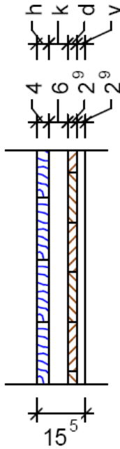
Wandtyp 15,5 horizontal
