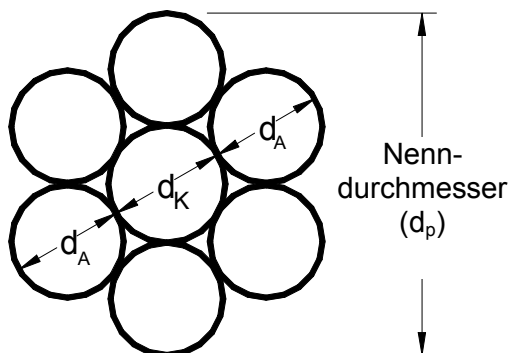
Bild 1 : Litzenquerschnitt
