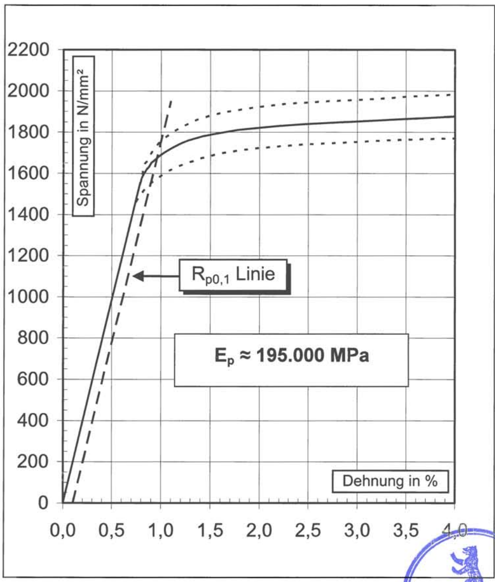
Bild 2: Spannungs – Dehnungslinie
