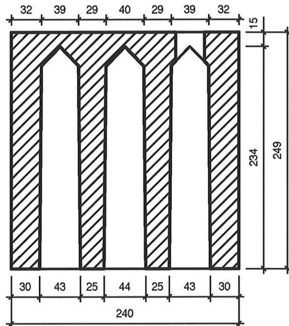
Schnitt A-A
