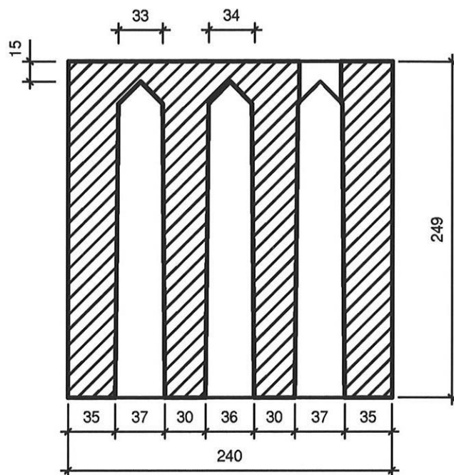
Schnitt A-A
