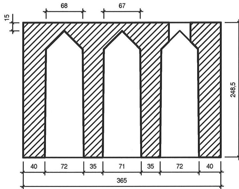
Untersicht
