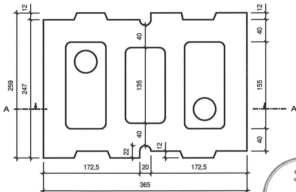
Untersicht
