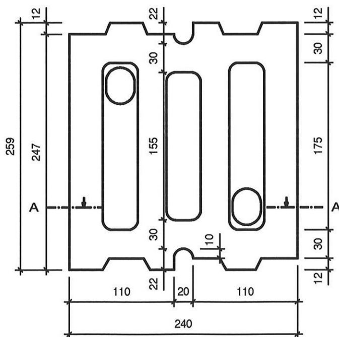
Untersicht
