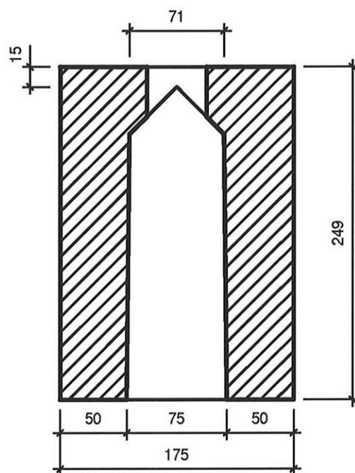
Schnitt A-A
