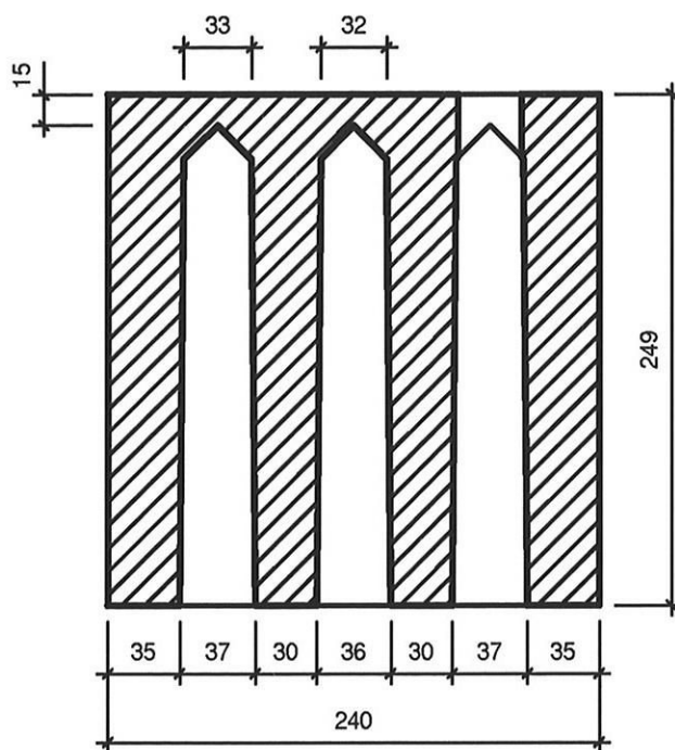
Schnitt A-A
