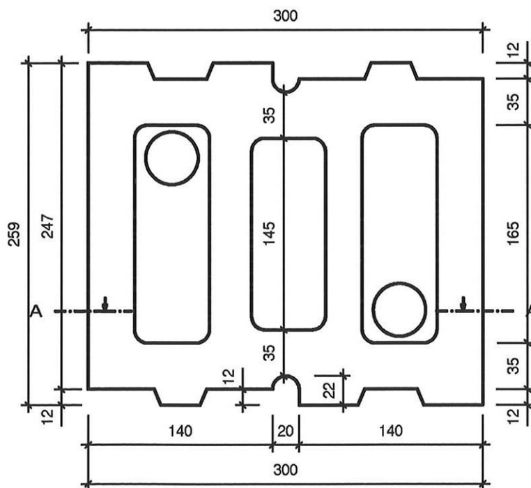
Untersicht
