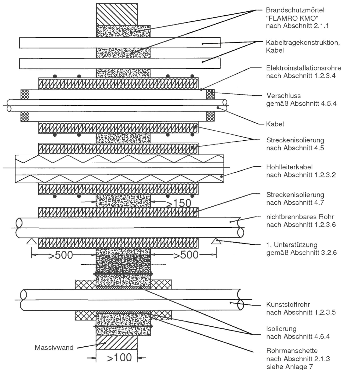
Schnitt A-A, B-B, und F-F
