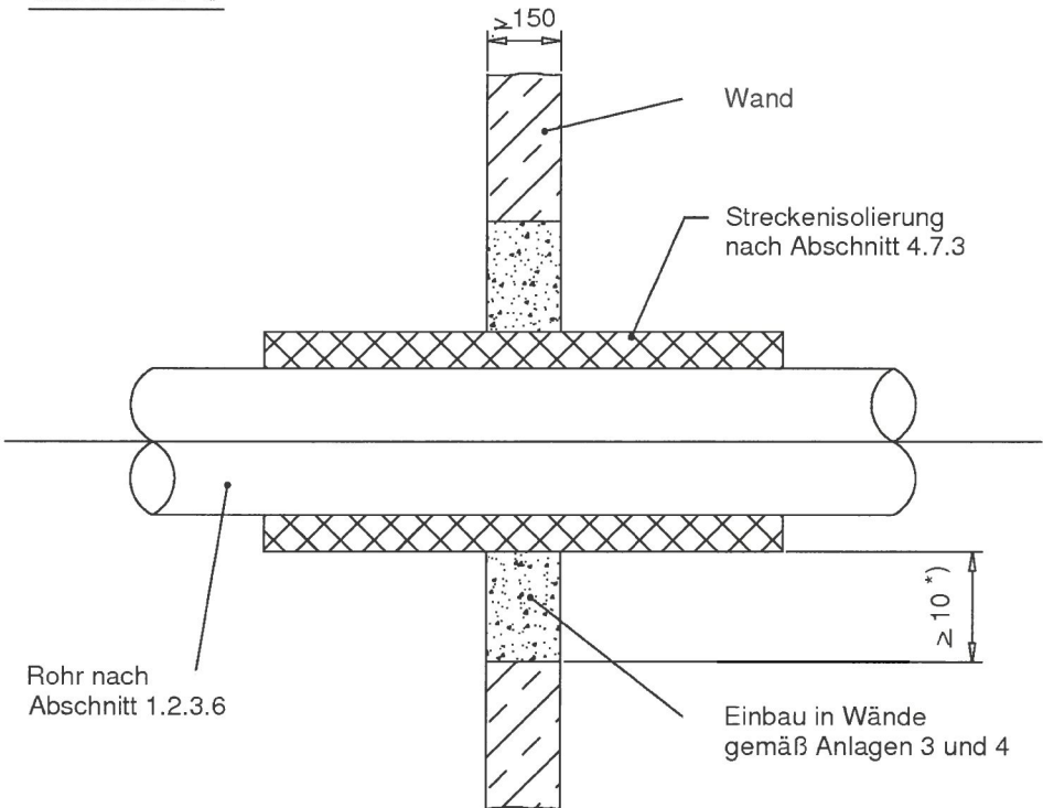
Schnitt J-J
