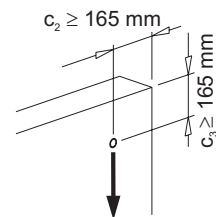
Bild 19: Einbausituation Wandfläche - Querbeanspruchung ohne Betonkantenbruch, ohne Rückhängebewehrung für Aufhängekonus 15,0 5cm und Sonderaufhängekonus R 3cm
