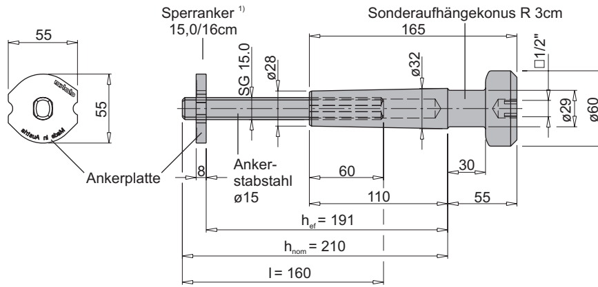
Bild 9: Sonderaufhängekonus R 3cm mit Sperranker 15,0 16cm
