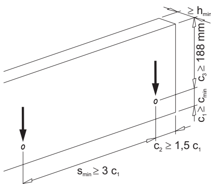
Bild 18: Einbausituation Wandfläche - Querbeanspruchung mit Betonkantenbruch, ohne Rückhängebewehrung
