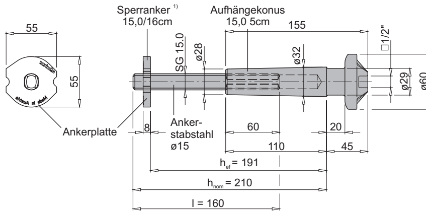
Bild 7: Aufhängekonus 15,0 5cm mit Sperranker 15,0 16cm
