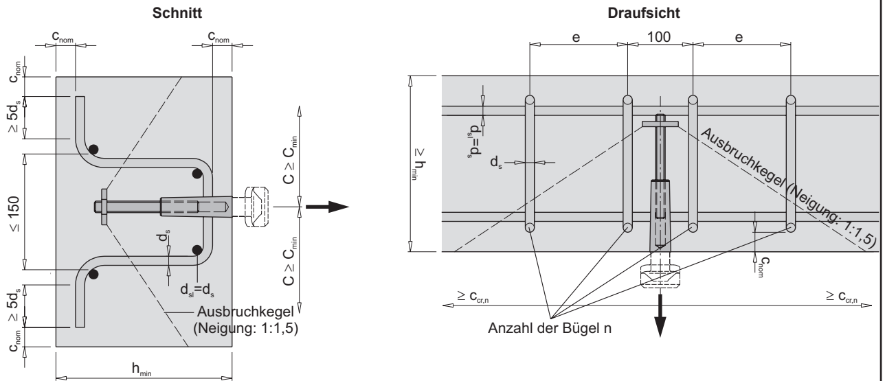
Bild 25: Einbausituation in dünne Wände - Zugbeanspruchung mit Rückhängebewehrung - Bewehrungslage
