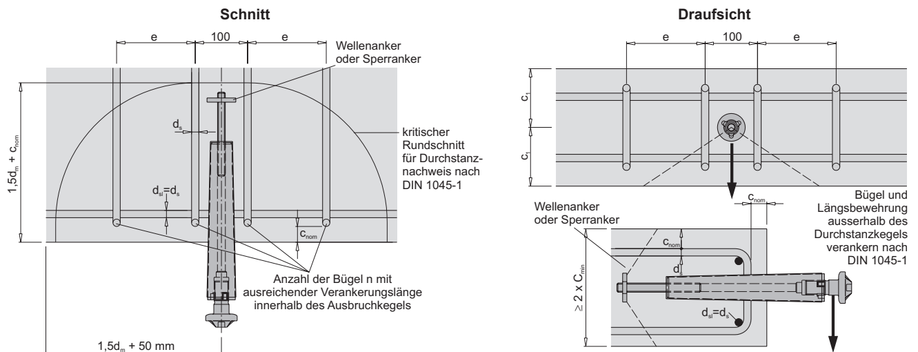
Bild 30: Einbausituation Stirnseite - Querbeanspruchung mit Rückhängebewehrung - Bewehrungslage
