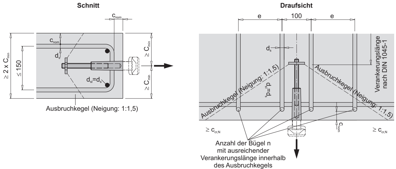
Bild 23: Einbausituation Stirnseite - Zugbeanspruchung mit Rückhängebewehrung - Bewehrungslage
