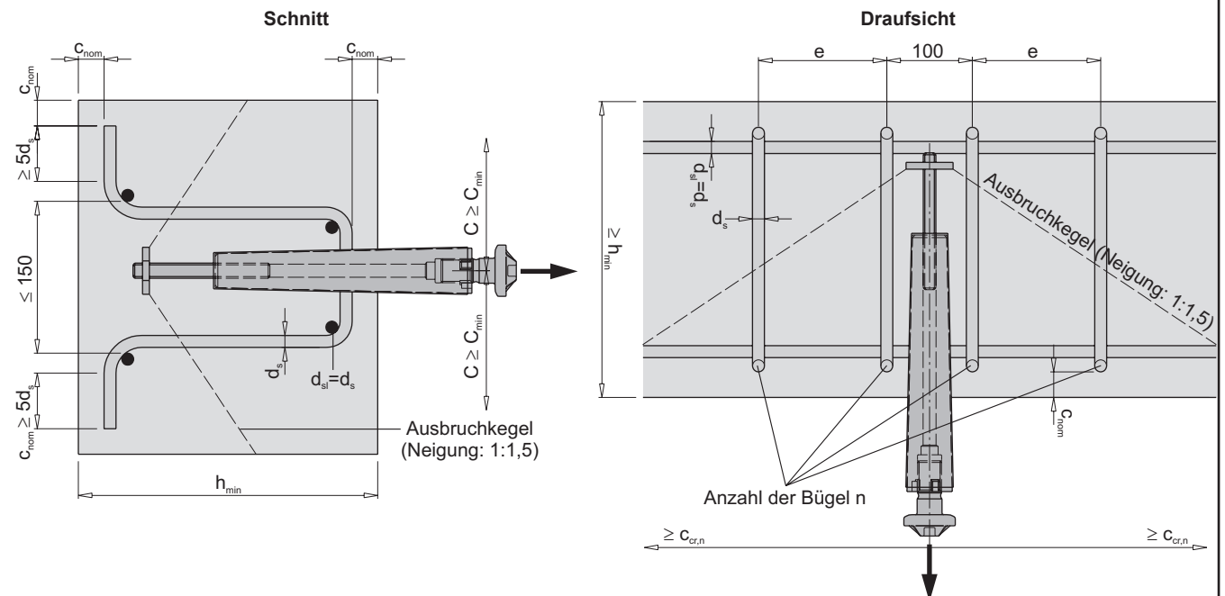
Bild 26: Einbausituation in dünne Wände - Zugbeanspruchung mit Rückhängebewehrung - Bewehrungslage
