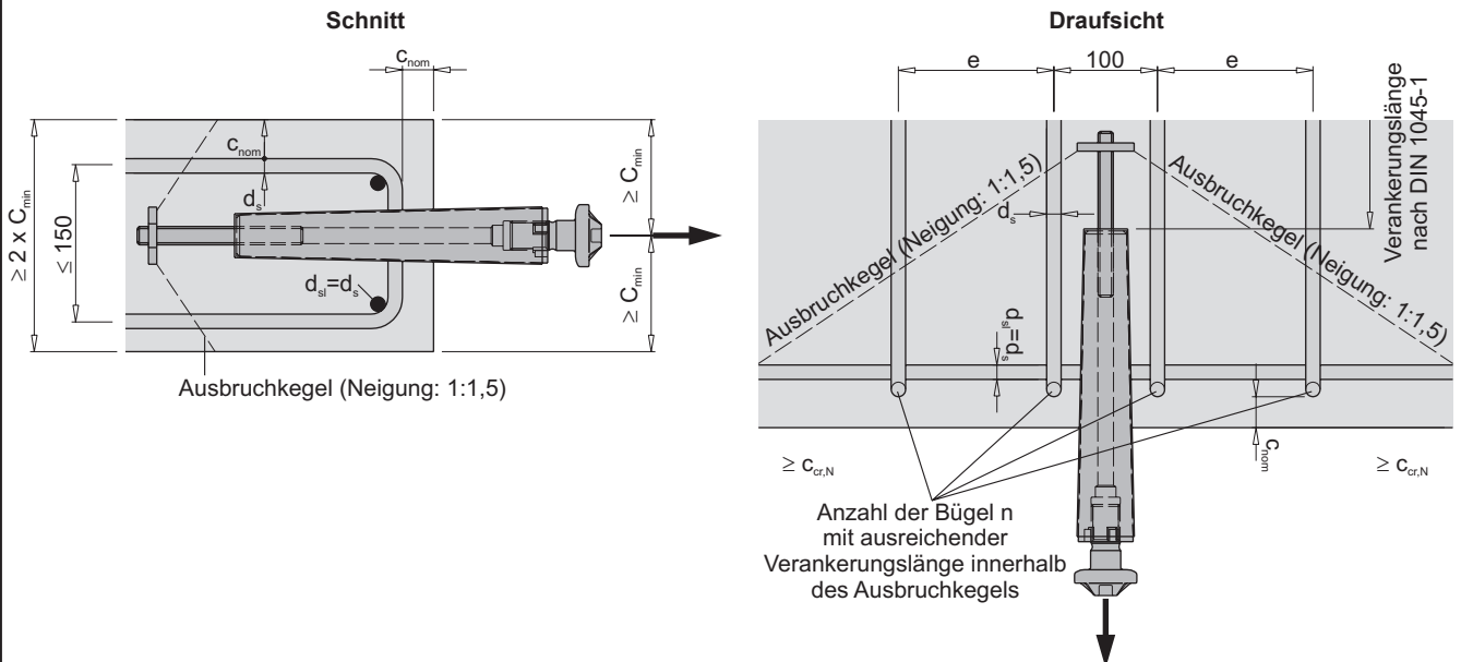
Bild 24: Einbausituation Stirnseite - Zugbeanspruchung mit Rückhängebewehrung - Bewehrungslage
