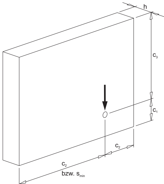
Bild 22: Randabstände bei Querbeanspruchung
