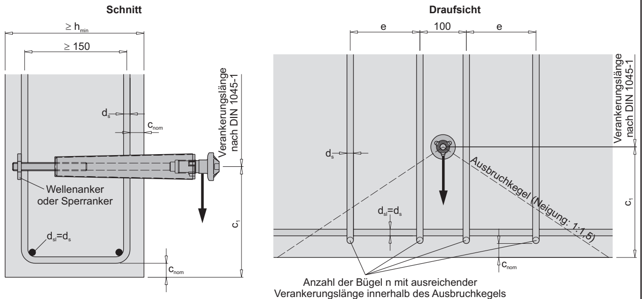
Bild 28: Einbausituation in Wänden - Querbeanspruchung mit Rückhängebewehrung - Bewehrungslage
