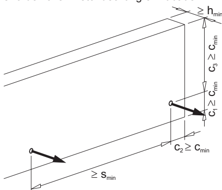
Bild 17: Einbausituation Wandfläche - Zugbeanspruchung, ohne Rückhängebewehrung
