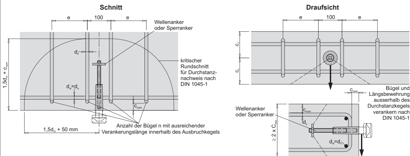
Bild 29: Einbausituation Stirnseite - Querbeanspruchung mit Rückhängebewehrung - Bewehrungslage
