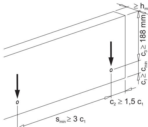
Bild 14: Einbausituation Wandfläche - Querbeanspruchung, ohne Rückhängebewehrung
