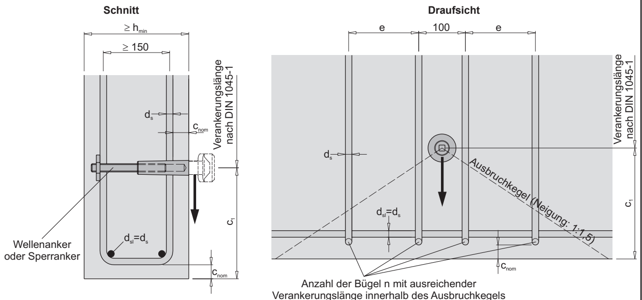
Bild 27: Einbausituation in Wänden - Querbeanspruchung mit Rückhängebewehrung - Bewehrungslage
