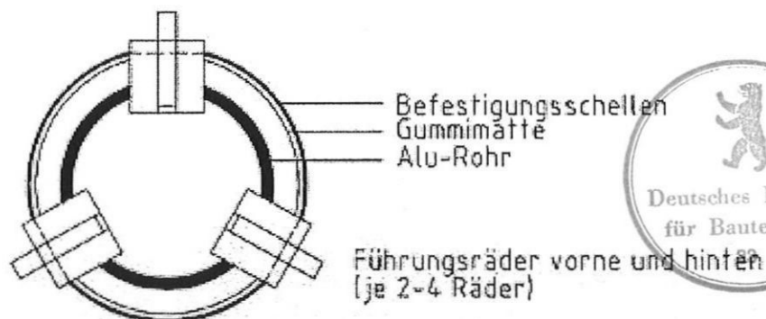
Ansicht Variante 1
