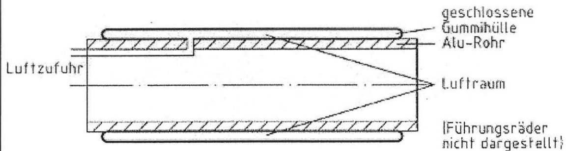
Längsschnitt
