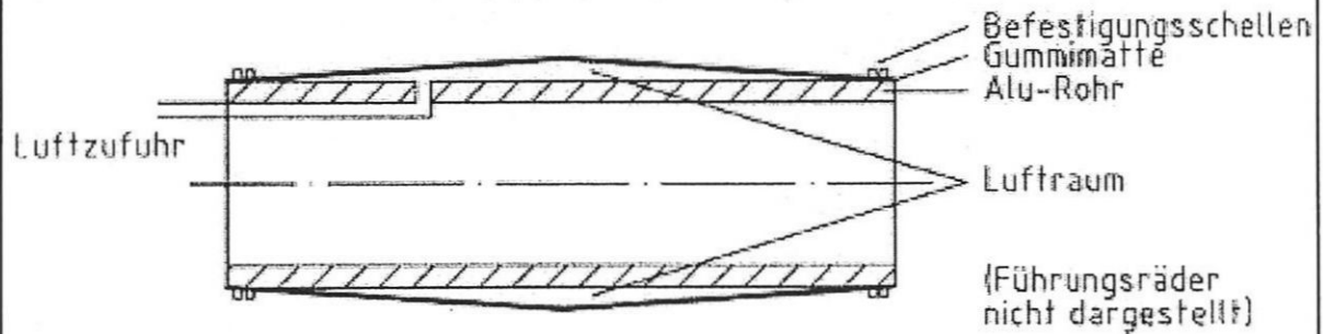
Längsschnitt
