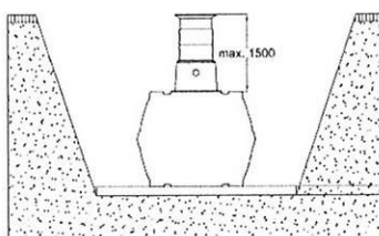
Überdeckungshöhen mit Zwischenstück und Teleskop Domschacht maximal (nur im Grünbereich ohne Grund- und Schichtenwasser)
