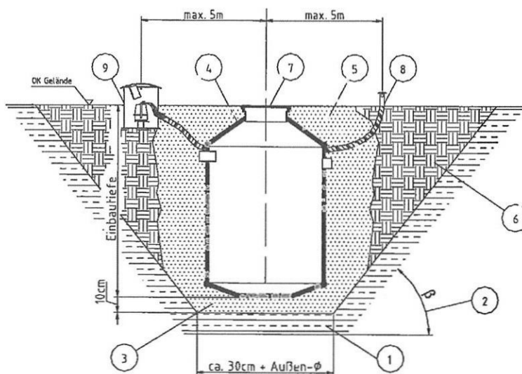
Einbaukskizze TORNADO Kleinkläranlage
