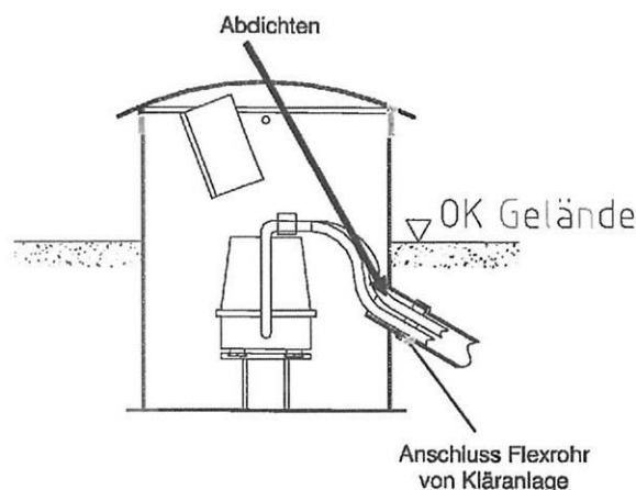
Einbauskeizze Außensteuersäule
