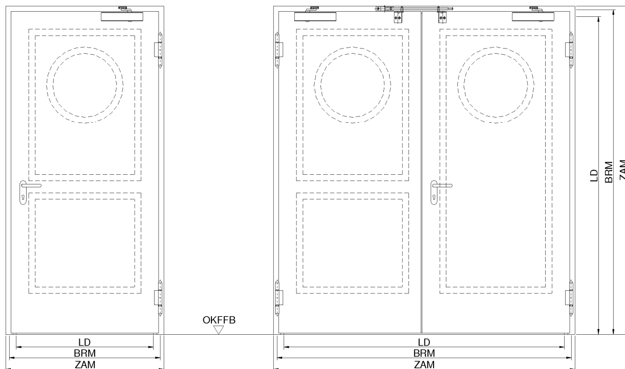
dargestellt: Anschlagrichtung DIN Rechts, DIN Links spiegelbildlich
